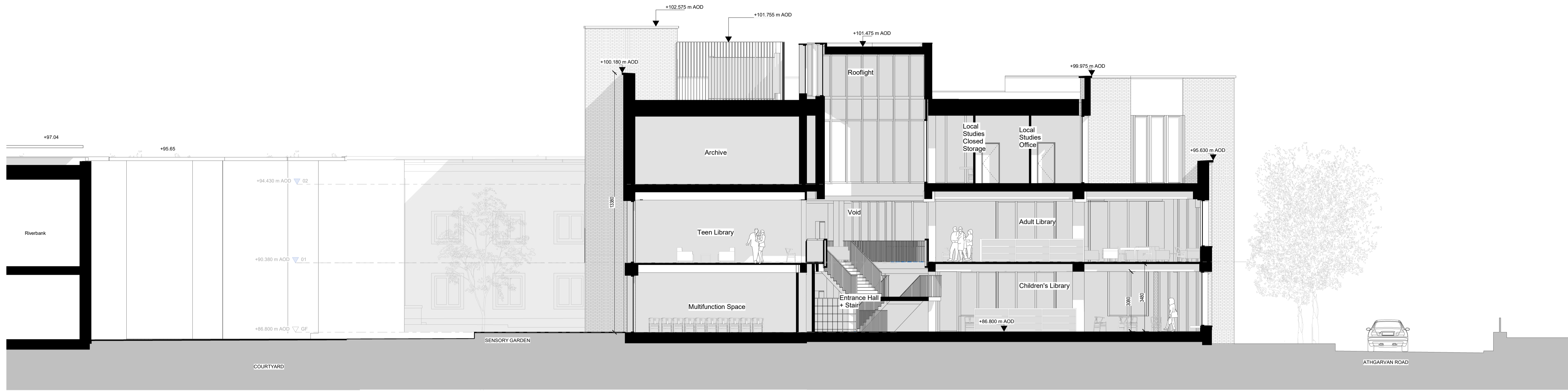
1. Section C-C 1 : 100
